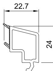
Lajsna za staklo 36 mm
