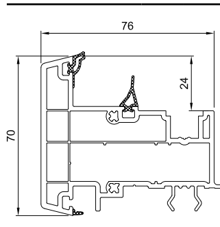
Lažna prečka 76 mm MD
