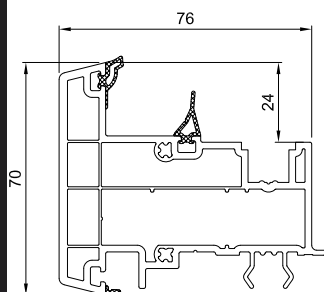
Lažna prečka 76 mm MD A klasa - Antracit spolja 6.5 m
