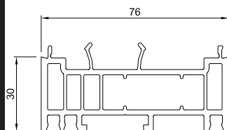
Proširenje 76x30 mm
