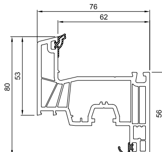
Krilo 76 mm MD - Antracit spolja A klasa / 6 komora 6.5 m
