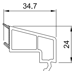
Lajsna za staklo 24 mm
