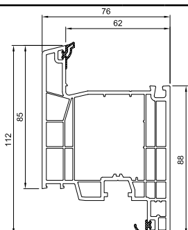
Krilo vrata 76 mm - Antracit
