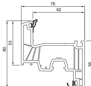
Krilo 76 mm MD - Zlatni hrast A klasa / 6 komora
