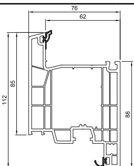
Krilo vrata 76 mm - Zlatni hrast Unutrašnje
