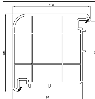
Skretnica 90° 76 mm
