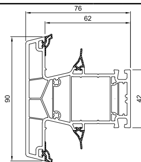
T prečka 76 mm MD A klasa - Antracit spolja 6.5 m
