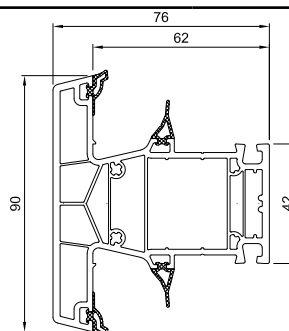
T prečka 76 mm MD - Antracit
