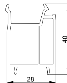
Podštok 28x40 mm
