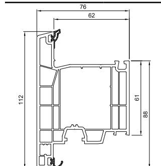
Krilo vrata 76 mm
