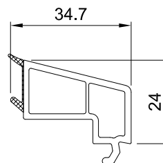
Lajsna za staklo 24 mm Zlatni hrast
