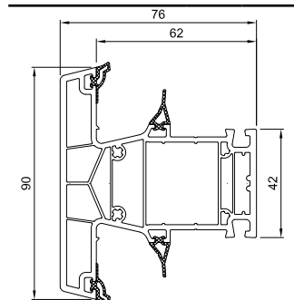
T prečka 76 mm MD
