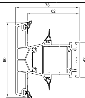
T prečka 76 mm MD A klasa - Zlatni hrast
