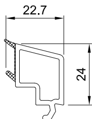
Lajsna za staklo 36 mm
