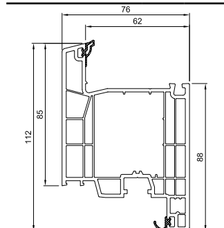
Krilo vrata 76 mm
