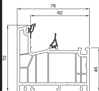
Štok 76 mm MD - Antracit spolja A klasa / 6 komora 6.5 m
