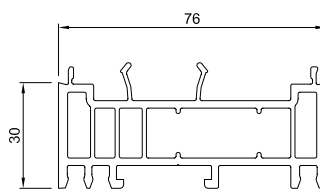
Proširenje 76x30 mm Antracit spolja 6 m
