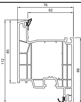
Krilo vrata 76 mm Unutrašnje - Antracit spolja 6.5 m
