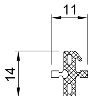
Spoj štokova
